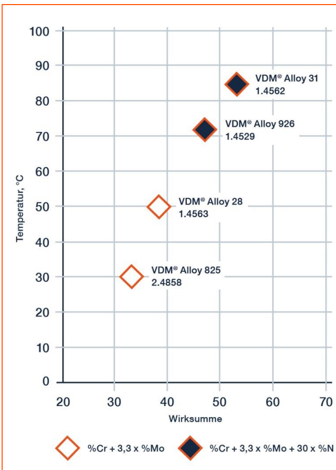
Abbildung 3 – Kritische Lochkorrosion (KLT) in 10 % FeCl 3 x 6 H 2 O als Funktion der entsprechenden Wirksummen; Bestimmung mit stufenweiser Temperaturerhebung unter Verwendung derselben Proben
