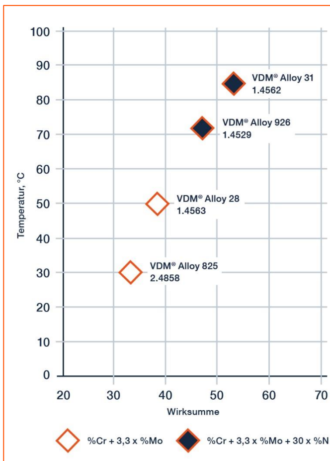
Abbildung 3 – Kritische Lochkorrosion (KLT) in 10 % \text{FeCl}_3 \times 6 \text{H}_2\text{O} als Funktion der entsprechenden Wirksummen; Bestimmung mit stufenweiser Temperaturerhebung unter Verwendung derselben Proben
